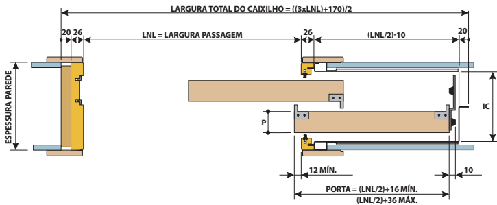
PARA 2 PORTA (dimensões em mm)
