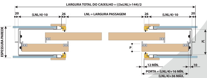
PARA 4 PORTAS (dimensões em mm)
