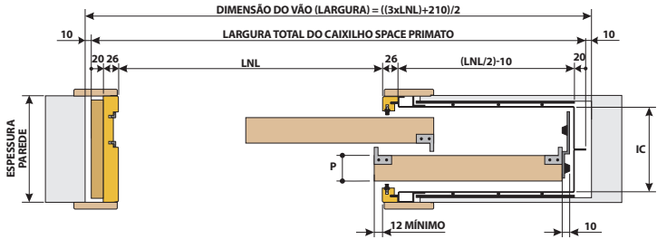
PARA 2 PORTAS (dimensões em mm)
