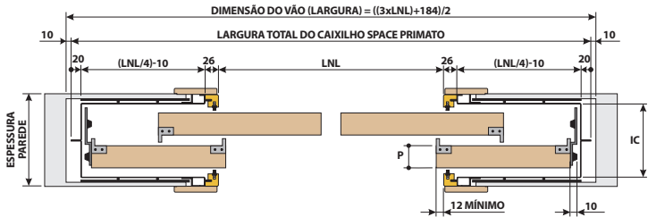
PARA 4 PORTAS (dimensões em mm)
